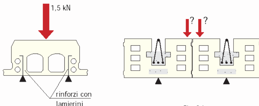
Figura 21. Esempio di blocco in polistirolo irrigidito da due lamierini: verifica della resistenza a punzonamento mediante carico concentrato 54 .
