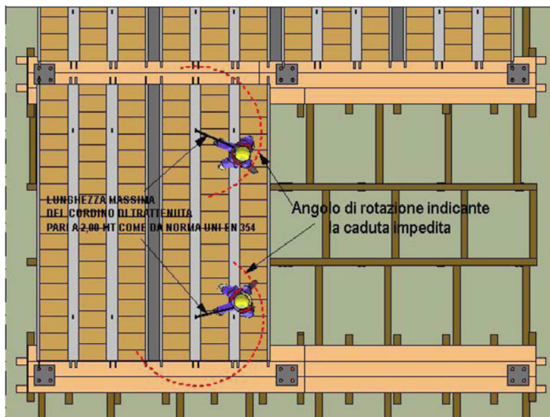
Figura 18. Schema di aggancio al pannello già posato con linea di ingombro del raggio d'azione del cordino a completa trattenuta 48 .
