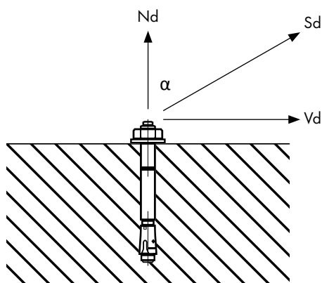
Fig. 7.1.2-1 Ancoraggio
