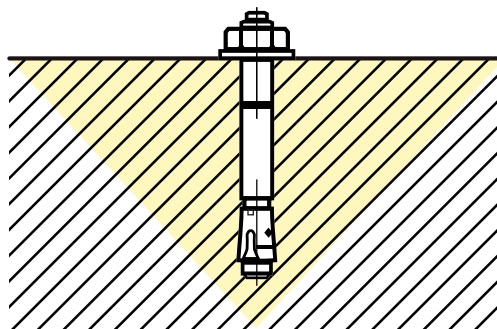
Fig. 7.1.3-7 Corretta scelta
